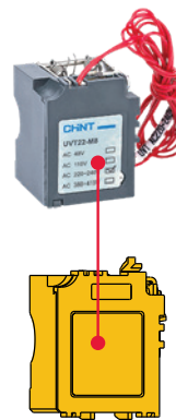
NM8N Underspennings-utløser 125A-630A
